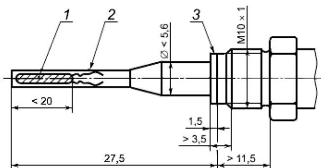
Рисунок 1 - Датчик температуры - тип DS
