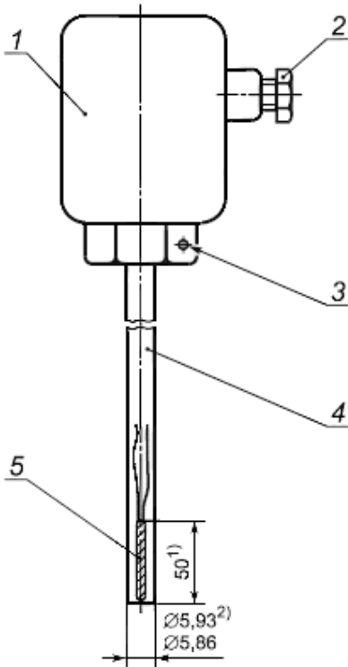
Рисунок А.4 - Датчик температуры, установка в гильзе, тип PL - головка
