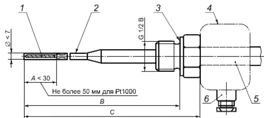
Рисунок 2 - Датчик температуры - тип DL (с головкой или кабелем)
