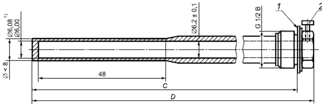
Рисунок 4 - Гильза датчика температуры
