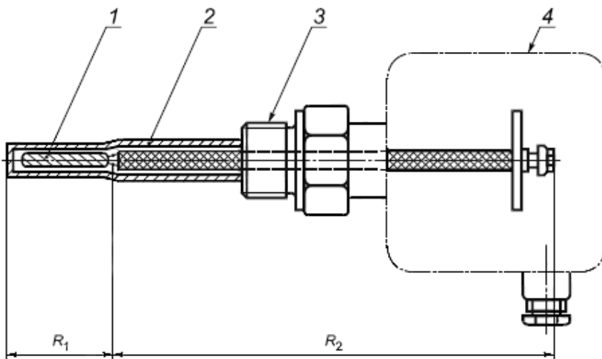
Рисунок 6 - Датчик температуры с соединительной головкой
