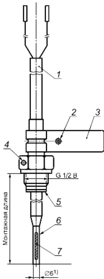
Рисунок А.3 - Датчик температуры, прямая установка, длинный, тип DL - кабель
