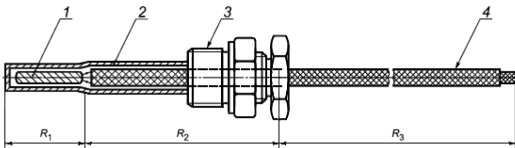
Рисунок 5 - Датчик температуры с постоянно присоединенным кабелем
