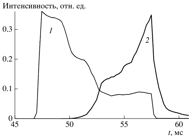
Рис. 1. Эволюция СВЧ-мощности – I , проходящей через слой порошковой смеси Fe + Al 2 O 3 толщиной 0.5 мм, и интенсивности интегрального оптического излучения разряда – 2. Начало СВЧ-импульса при t = 47 мс.
