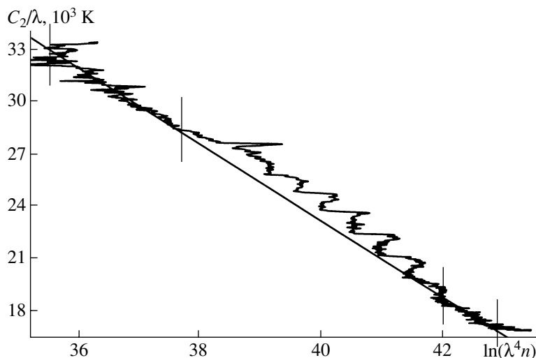
Рис. 7. Спектр излучения СВЧ-разряда в планковских координатах для порошка \text{SrO}_3 . Вертикальные отрезки ограничивают диапазоны ( \lambda = 430\text{--}500 и \lambda = 750\text{--}840 нм), по которым проводилось определение температуры ( T \approx 2185 К).
