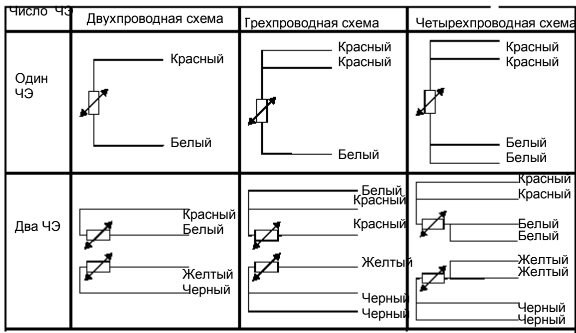
Рисунок 1 – Схемы соединения внутренних проводов
